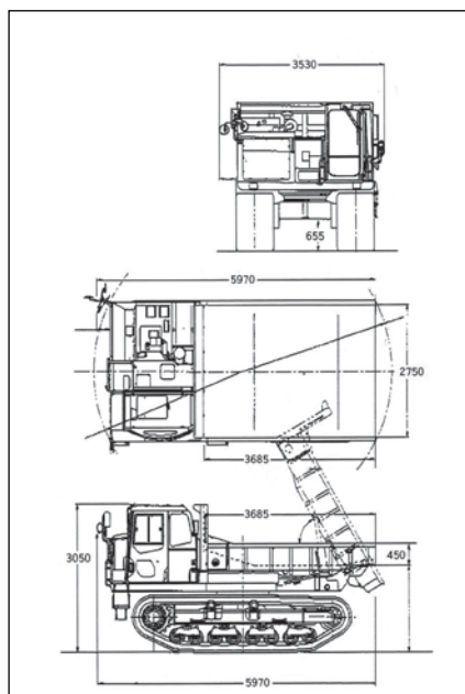
CD110R-1 外形寸法(mm)
