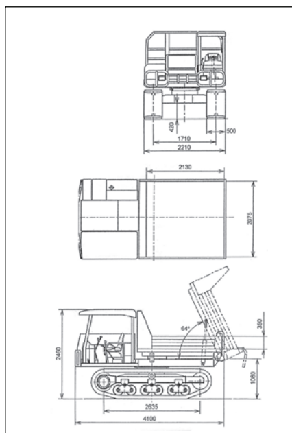
MST-800VT 外形寸法(mm)
