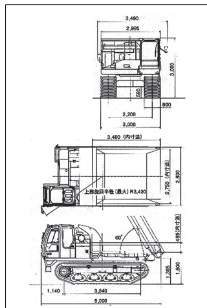
EG110R 外形寸法(mm)
