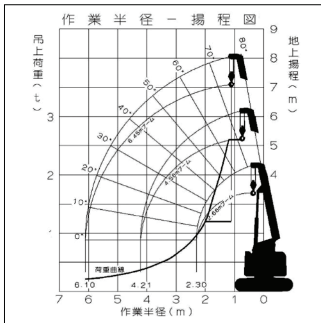
CX26-3 定格総荷重(4本掛け時)
