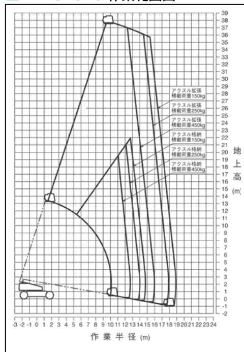
AW-370TG 作業範囲図
