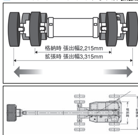
AW-250TG/AW-370TG アクスル拡張図
