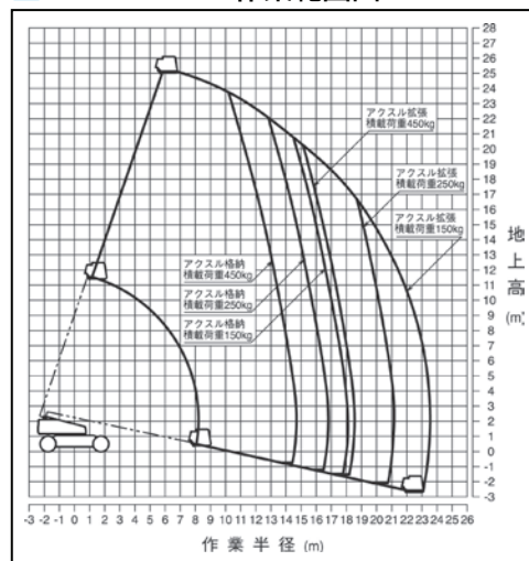
AW-250TG 作業範囲図
