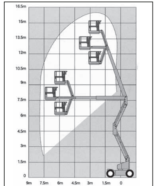
AB46E 作業範囲図
