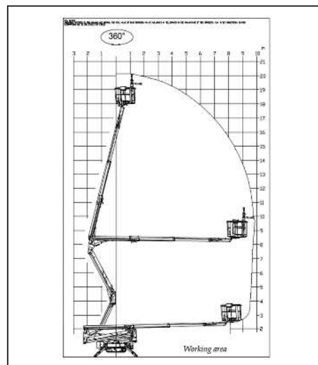
■ X20J PLUS 作業範囲図
